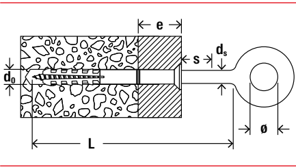
Golfare per ponteggi GS Ø23 mm
